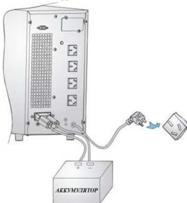
Рисунок 3.3 - Схема подключения аккумуляторов для моделей с увеличенным временем автономной работы
